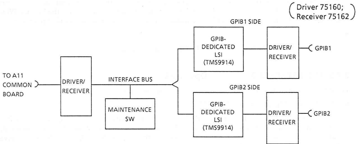
Fig. 2-19 A7 Interface 1
